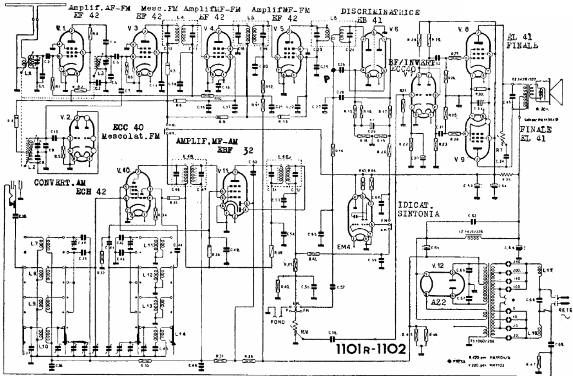
S.A. FIMI - Mod. PHONOLA 1101 R e 1102 - A modulazione d'ampiezza e di frequenza. Onde medie divise e sei bande allargate ad onde corte. Medie frequenze: AM 470 kc, FM 10,5 Mc. (Valori v. Tabella a parte).
